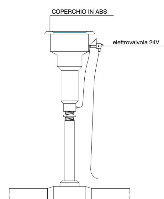
PARTICOLARE IRRIGATORE CON ELETTROVALVOLA INCORPORATA "RAIN BIRD" mod. EAGLE - 950 - E/28
