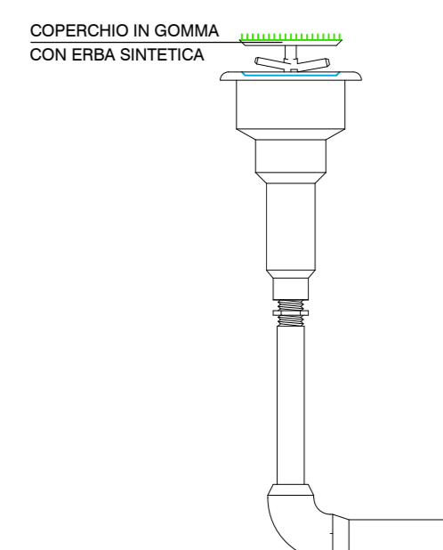
PARTICOLARE IRRIGATORE A TURBINA "RAIN BIRD" mod. EAGLE - 900 - E/30
