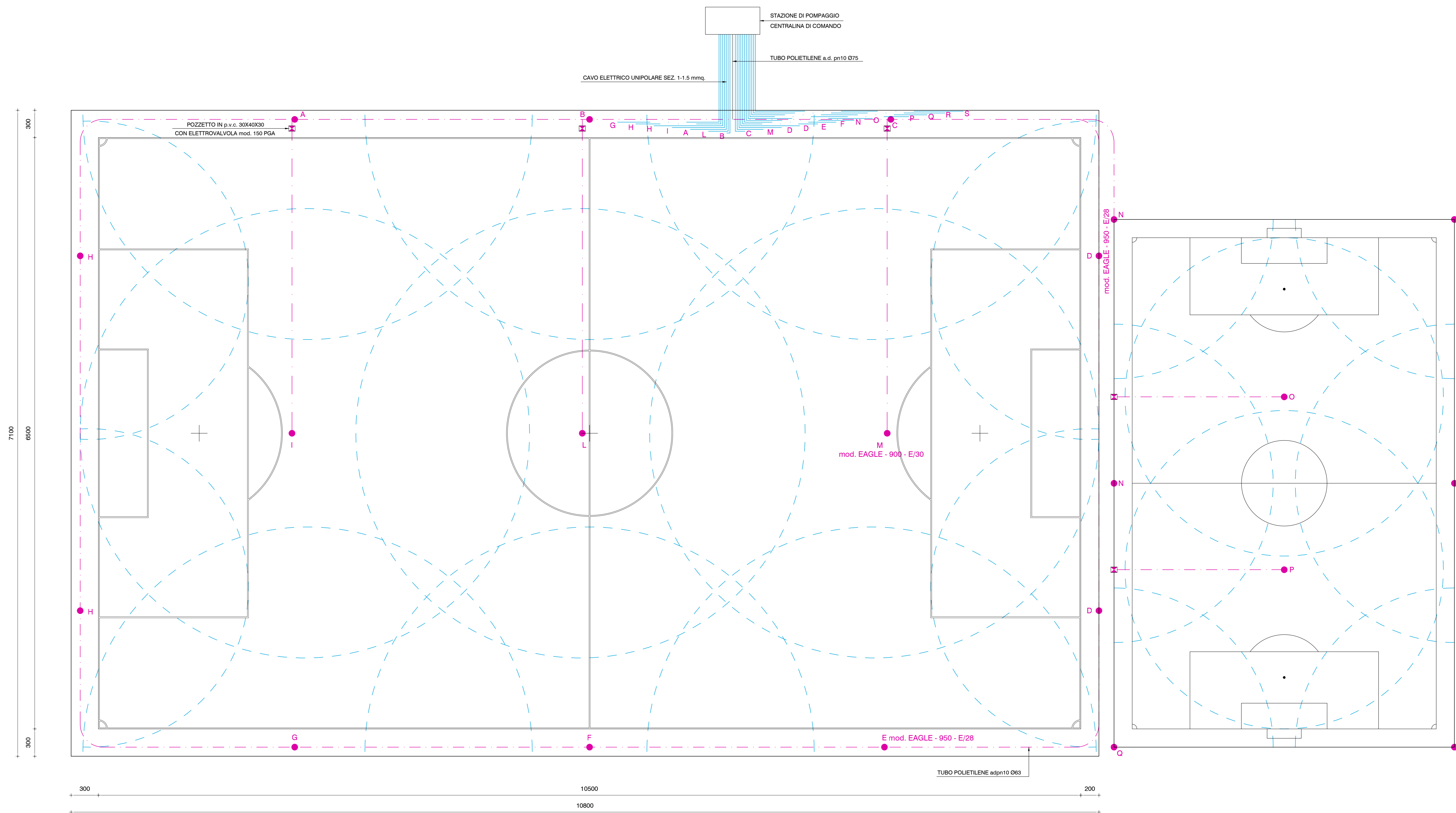
PLANIMETRIA IMPIANTI DI IRRIGAZIONE E ILLUMINAZIONE scala 1:200
